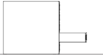
Seitenansicht orgaBox large und small 33,5 cm tief
